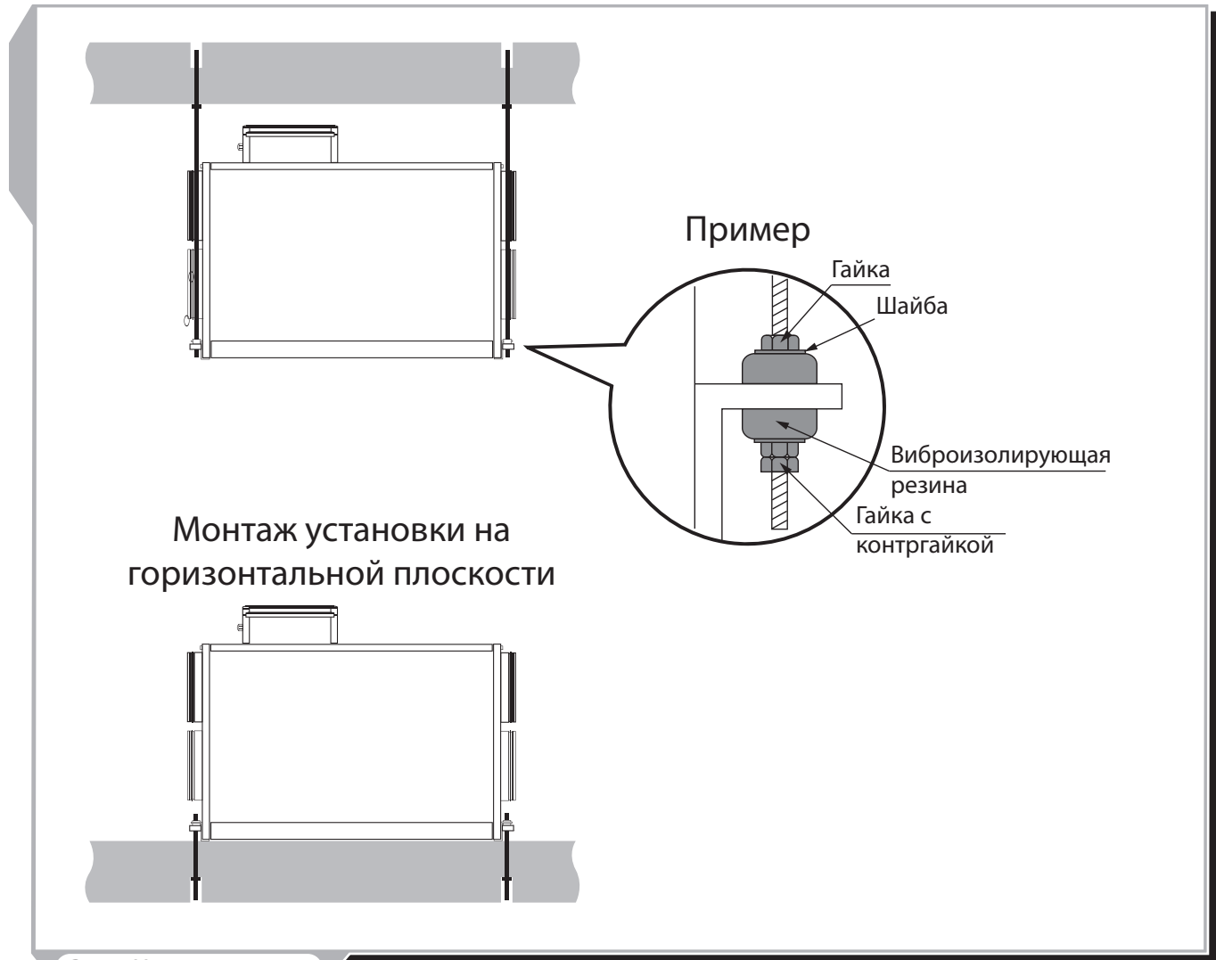
Рис. 5. Монтаж установки
