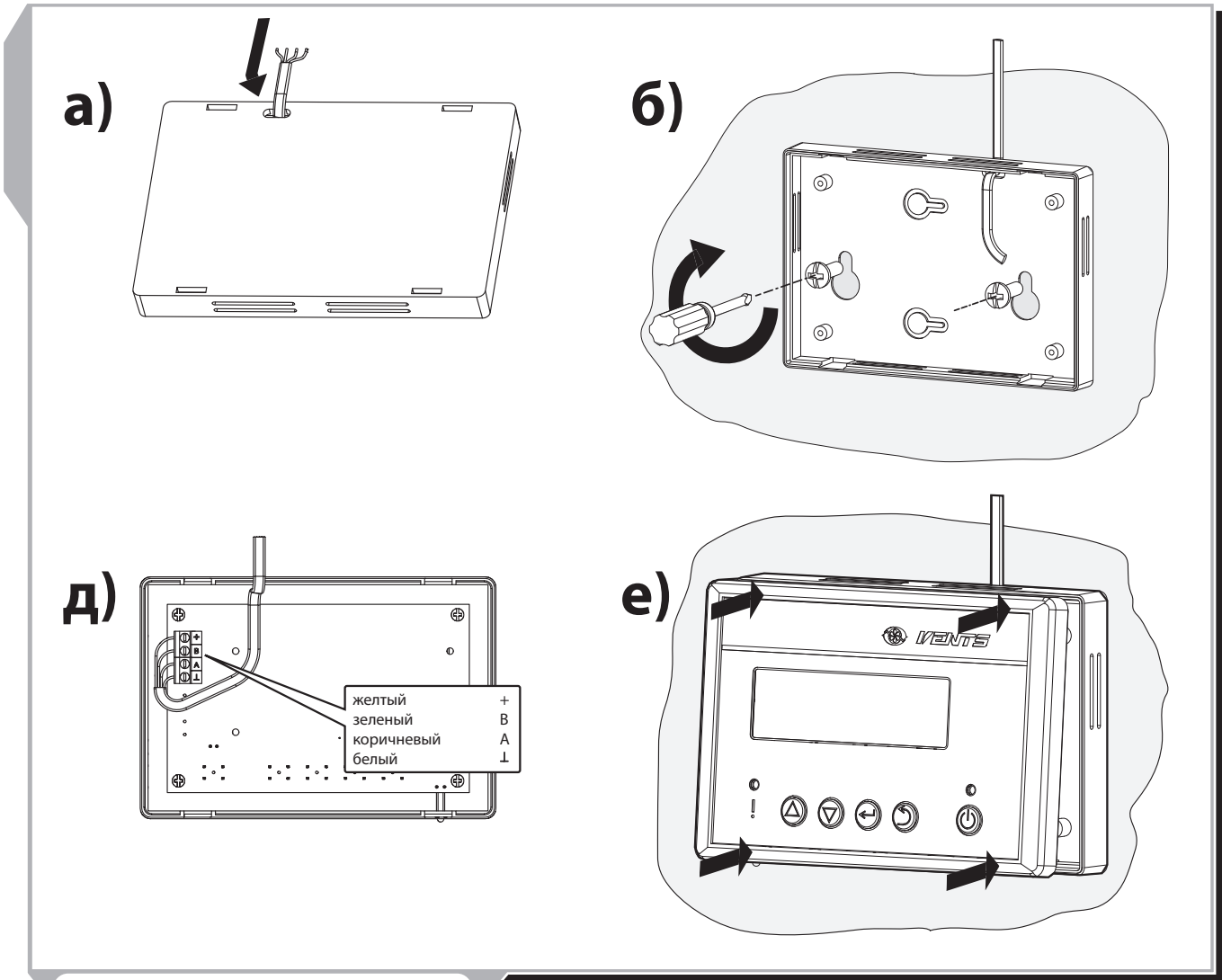
Рис. 10. Подключение пульта управления
