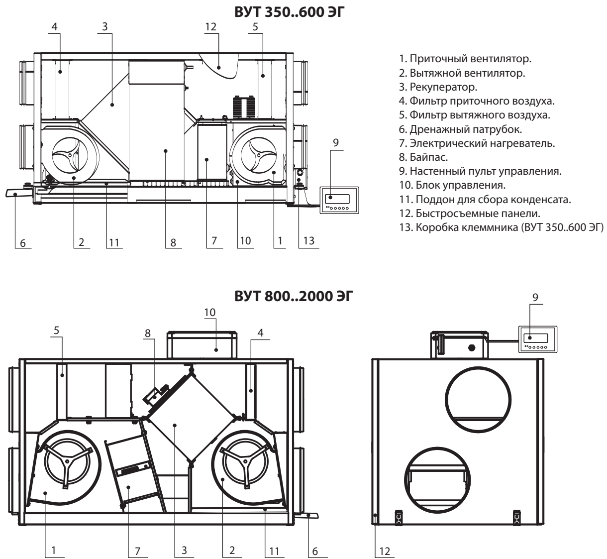
Рис. 4. Устройство установок
