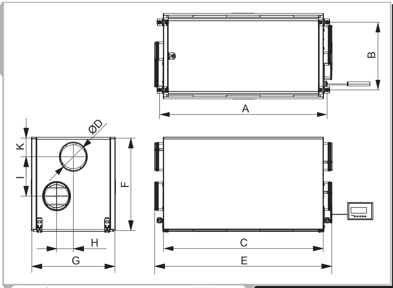
Рис. 1. Габаритные и присоединительные размеры для ВУТ ЭГ 350..600
